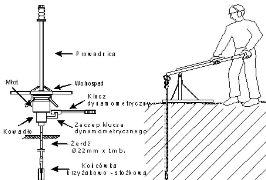
Lekka sonda udarowo-obrotowa typu SLVT do kompleksowych badań gruntu i wyciąg dźwigniowy do żerdzi
