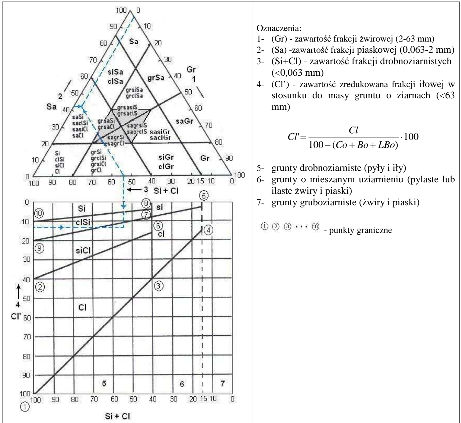
Trójkąt klasyfikacyjny z diagramem PN-EN ISO 14688
